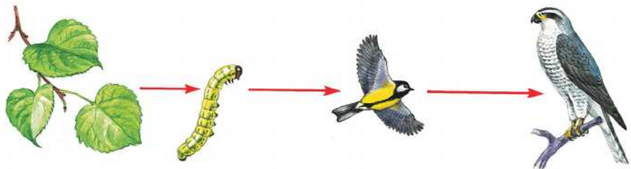
Рис. 71. Пищевая цепь
